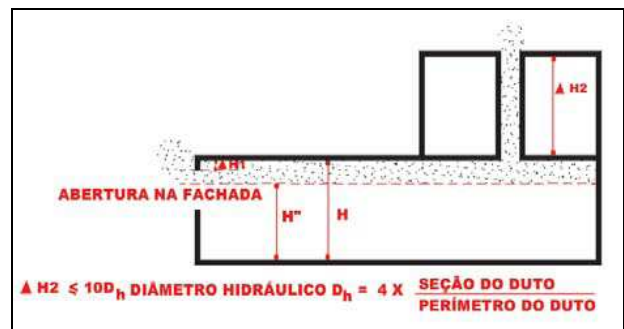
Figura 17: Diâmetro hidráulico
